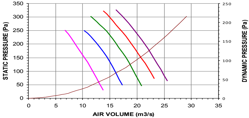
AF24-1400-5 RPM 720 20 °C
