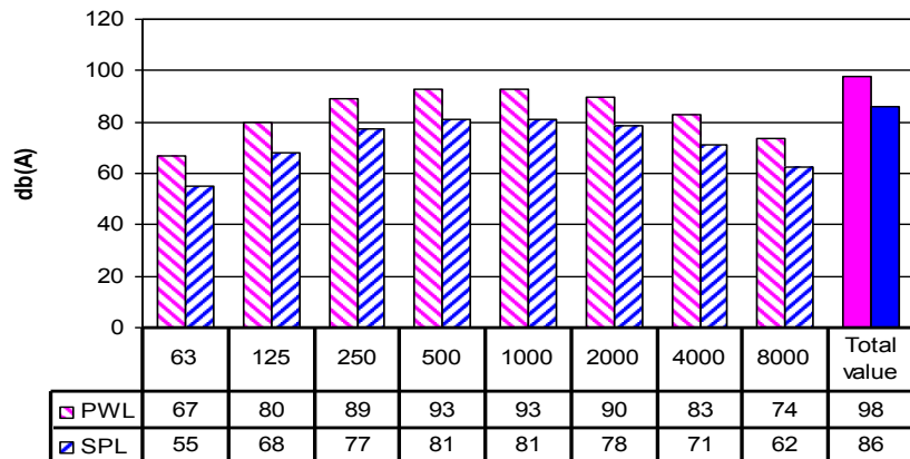
AF24-1400-5 RPM 720 20 °C
