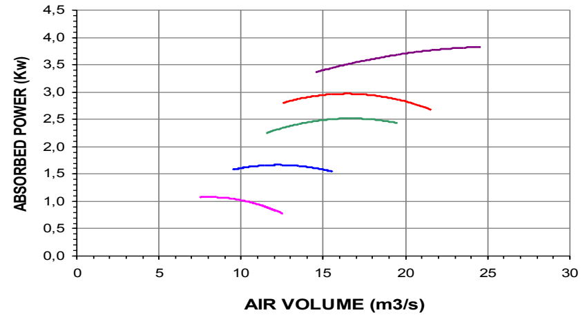
AF24-1600-4 RPM 480 20 °C
