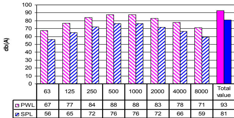
AF24-1600-4 RPM 480 20 °C
