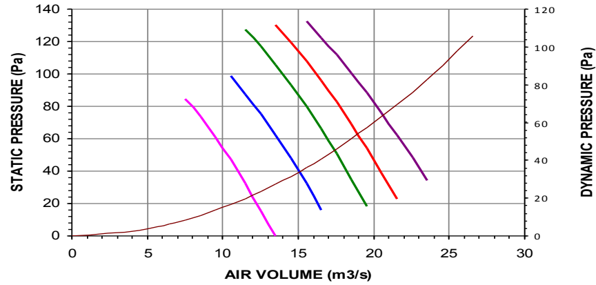
AF24-1600-4 RPM 480 20 °C
