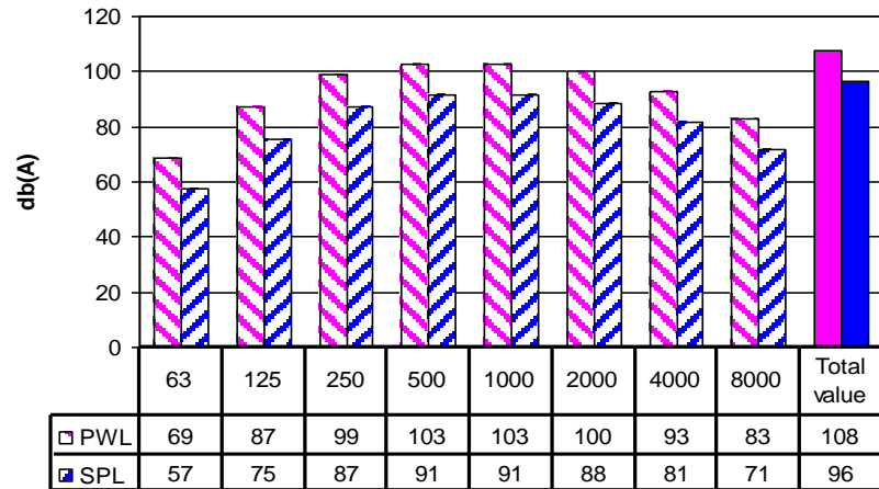
AF24-1600-9 RPM 960 20 °C
