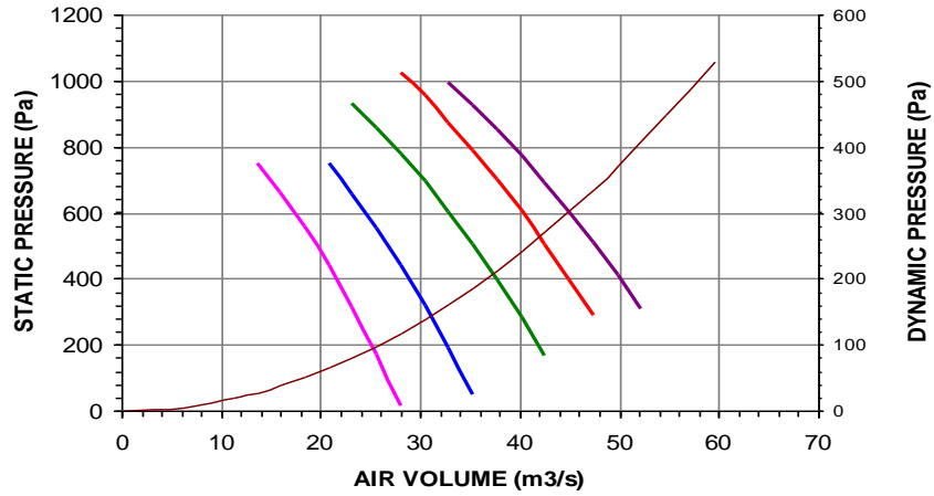
AF24-1600-9 RPM 960 20 °C
