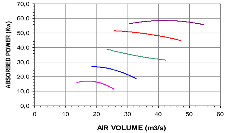
AF24-1600-9 RPM 960 20 °C
