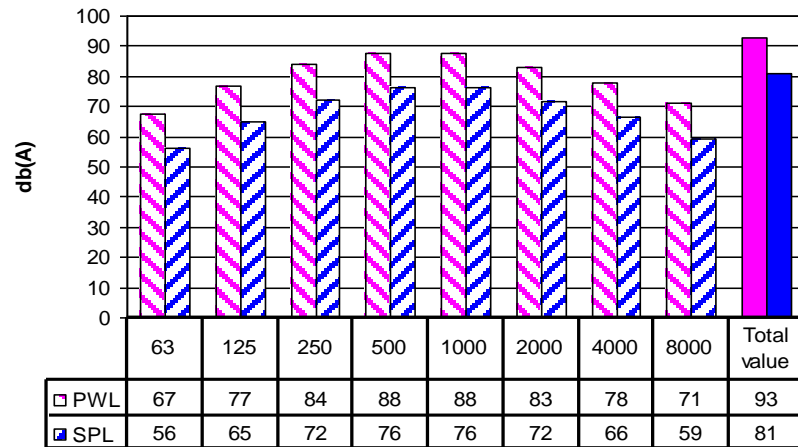
AF24-1600-4 RPM 480 20 °C
