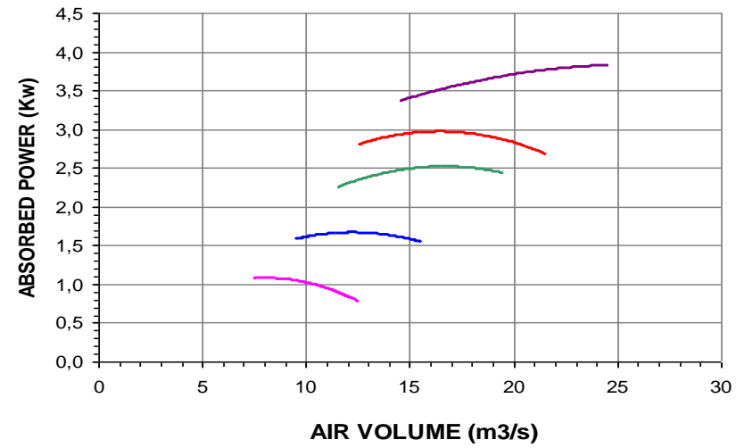
AF24-1600-4 RPM 480 20 °C
