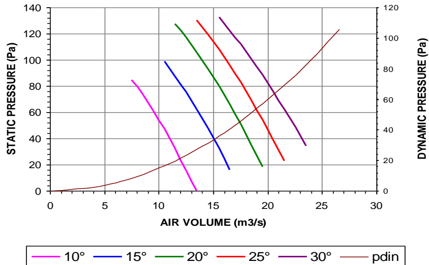
AF24-1600-4 RPM 480 20 °C
