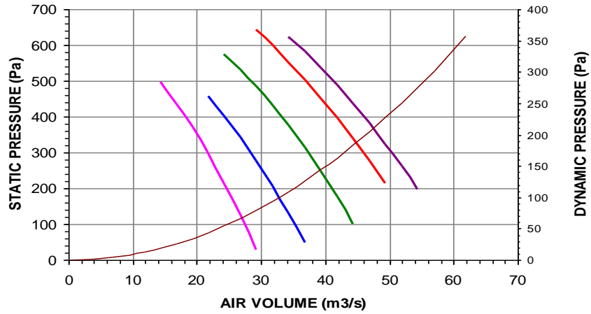
AF24-1800-8 RPM 720 20 °C
